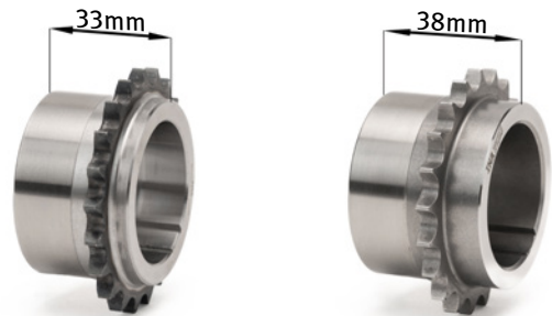
Bild 1: Das Kurbelwellenzahnrad 554 0996 10 mit einer Länge von 33mm (links) ist Bestandteil vom Steuerkettensatz 559 1780 30. Das Kurbelwellenzahnrad 554 0101 10 mit einer Länge von 38mm (rechts) ist Bestandteil vom Steuerkettensatz 559 1780 31
